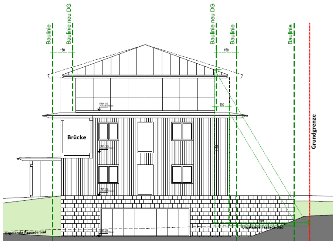
Abbildung 8: Gebäudeschnitt in Ost-West-Richtung (Quelle: Architekten Ronacher ZT GmbH)
